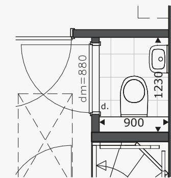
1 e verdieping
