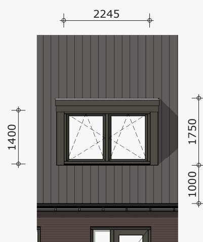
achtergevel
