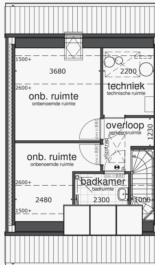
1 e verdieping
